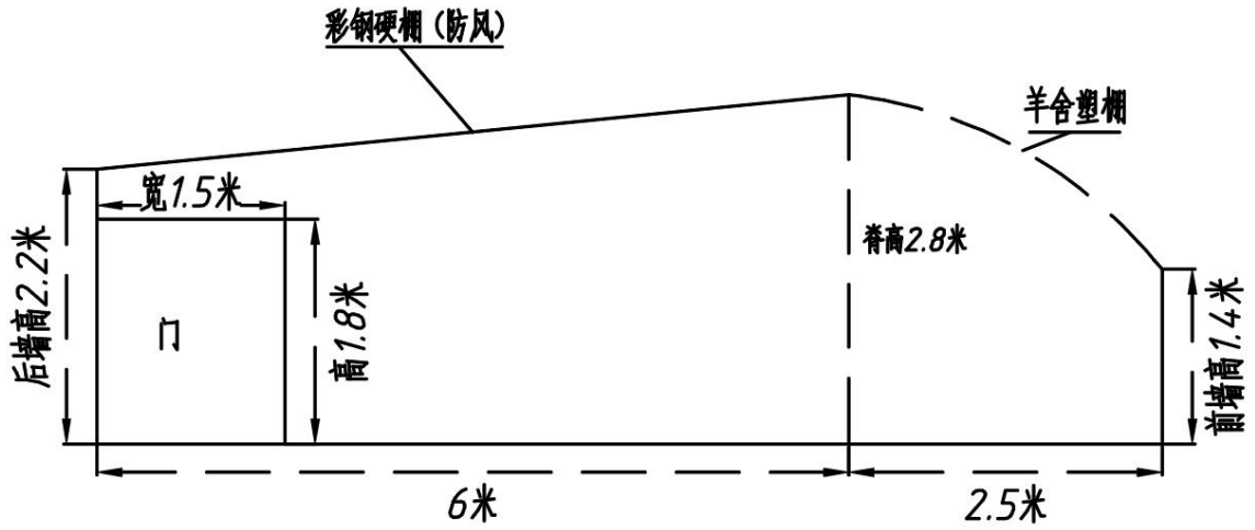
羊舍横切面图
